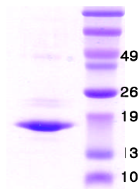
14% SDS-PAGE
