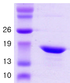
14% SDS-PAGE
