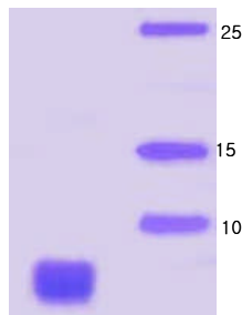
15% SDS-PAGE
