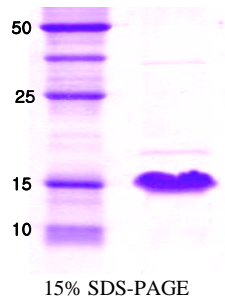
15% SDS-PAGE
