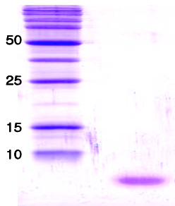
15% SDS-PAGE
