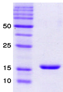
14% SDS-PAGE
