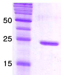
14% SDS-PAGE
