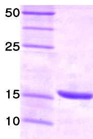
14% SDS-PAGE
