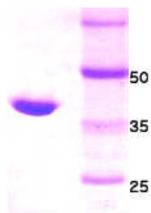
15% SDS-PAGE
